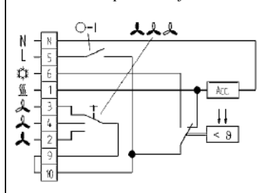
KLR-E 7009 kapcsolási rajza:
