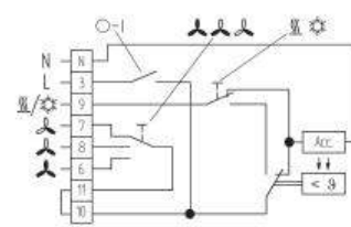
KLR-E 7010 kapcsolási rajza:
