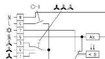
KLR-E 7011 kapcsolási rajza:
