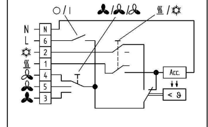
KLR-E 7012 kapcsolási rajza:
