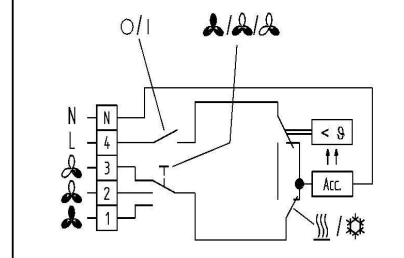
KLR-E 7015 kapcsolási rajza:
