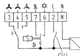
KLR-E 7203 kapcsolási rajza:
